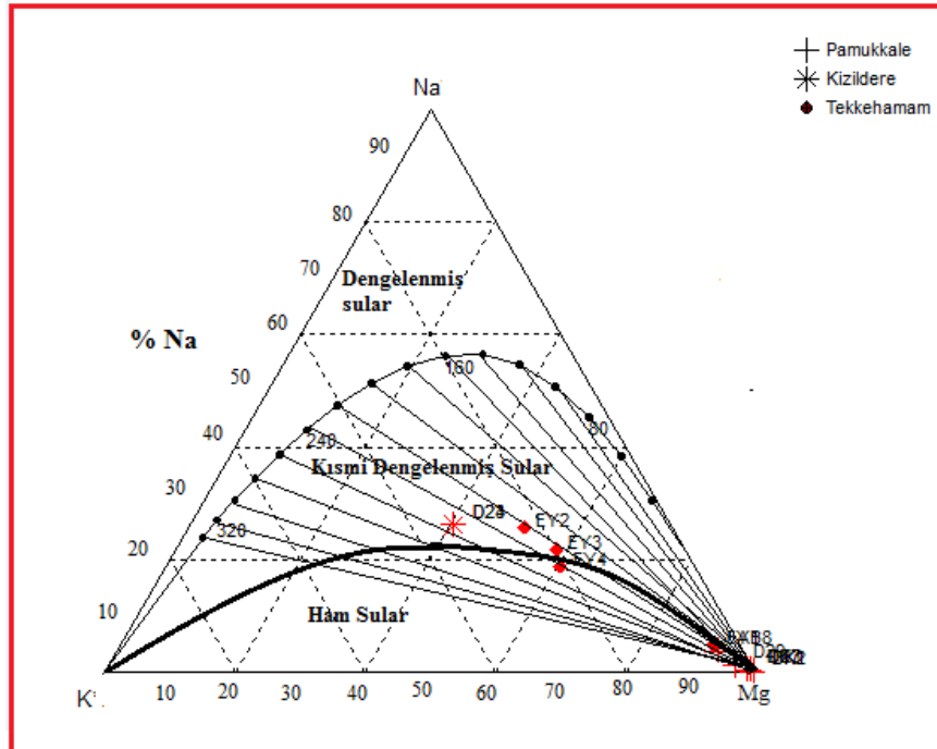
Şekil 5. 4. İnceleme alanındaki suların Na-K-Mg diyagramındaki görünümü ve su-kayaç denge sıcaklıkları (Giggenbach, 1988)
