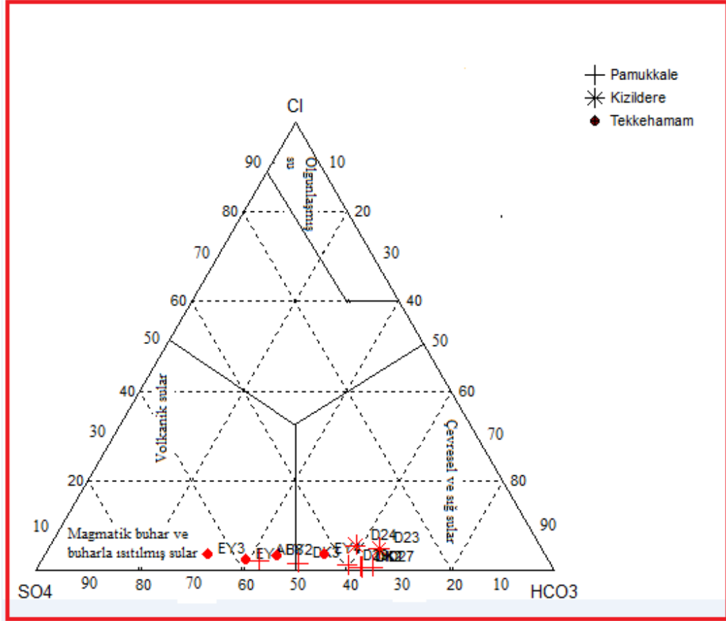
Şekil 5. 2. Tekkehamam ve çevresi jeotermal sularının Cl-SO 4 -HCO 3 üçgen diyagramı
